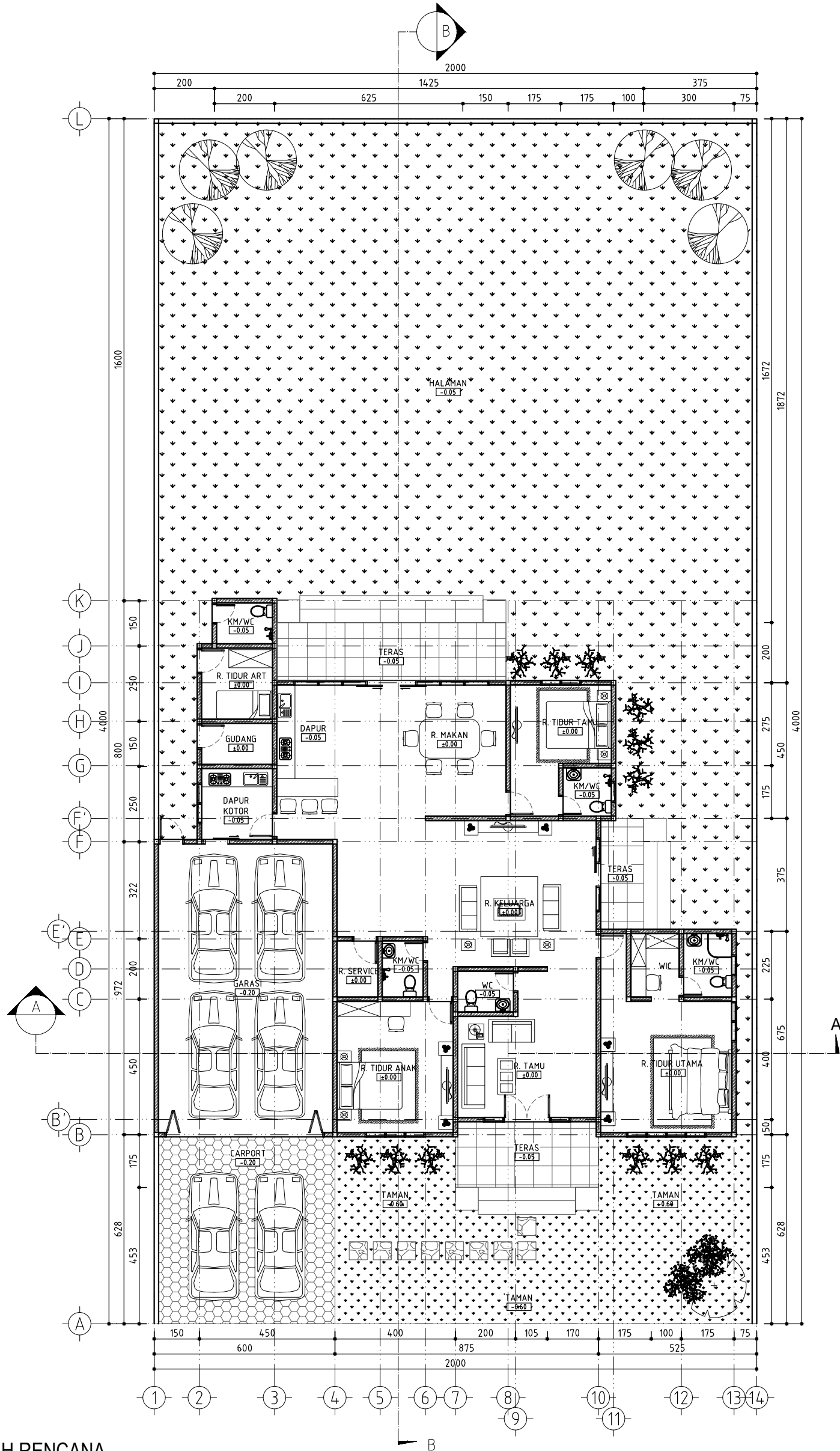
DENAH RENCANA SKALA 1 : 150
